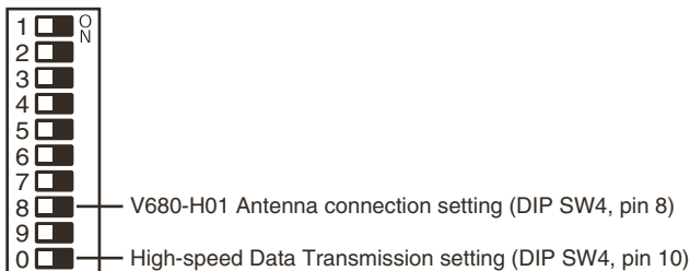
DIP SW4
