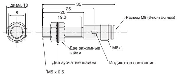
Рис. 36 : E2E-X1□□-M5
