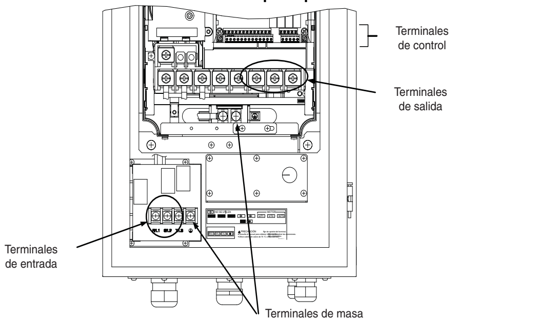
Fig. 3 Disposición de terminales de los variadores de 7,5 a 30 kW
