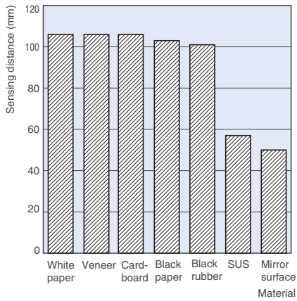
E3ZM-LS□1H(LS□6H)
