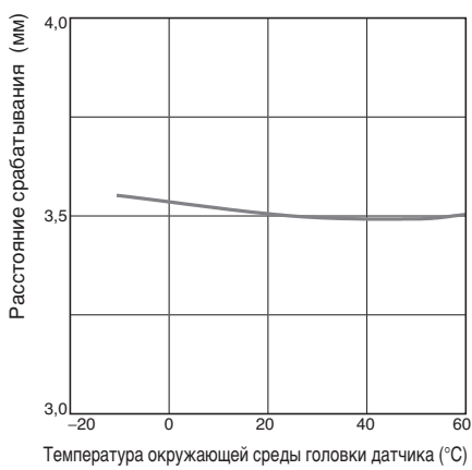
E2C-EM07(-□)
