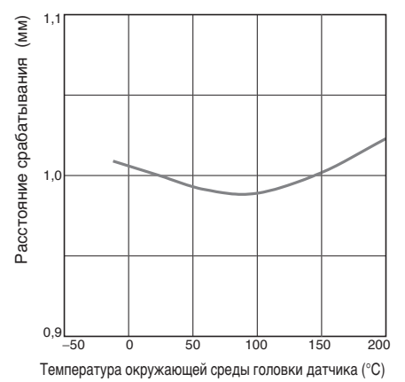
E2C-EM02H
