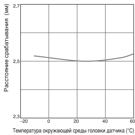
E2C-EV05(-□)
