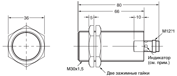
E2AU-M30LS15-M1-□□
