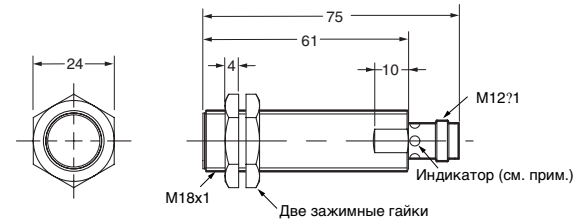
E2AU-M18LS08-M1-□□
