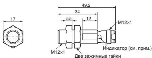
E2A3-M12KS06-M1-□□
