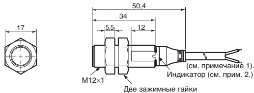
E2A3-M12KS06-WP-□□
