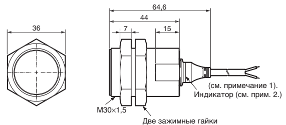
E2A3-M30KS20-WP-□□
