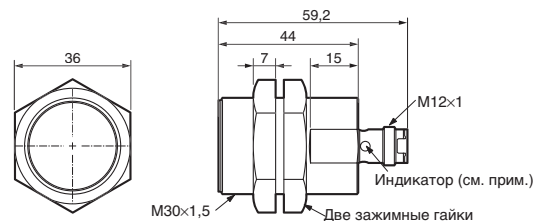
E2A3-M30KS20-M1-□□
