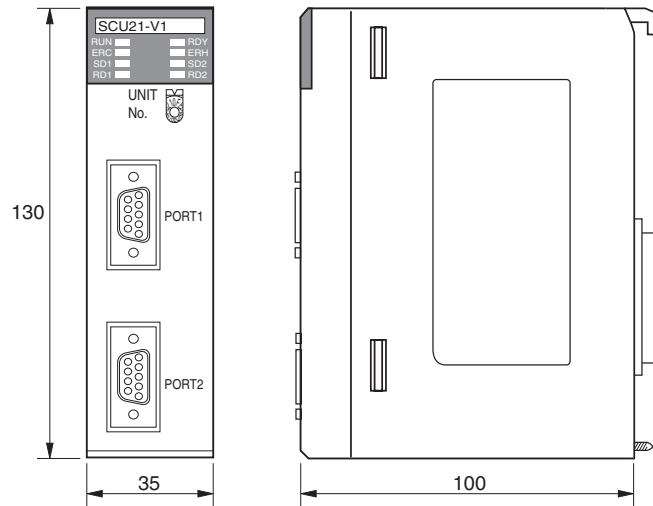
CS1W-SCU21-V1
