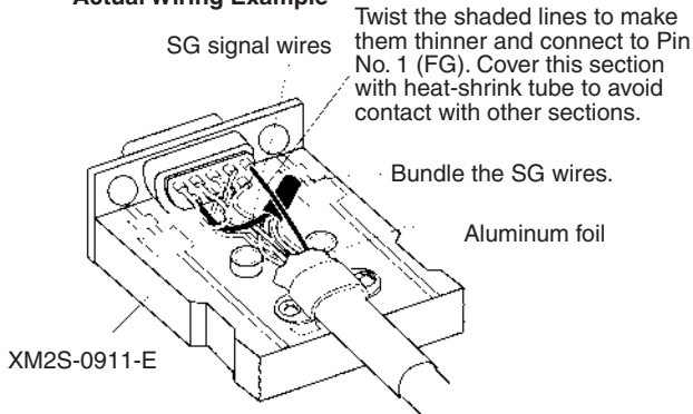
Actual Wiring Example
