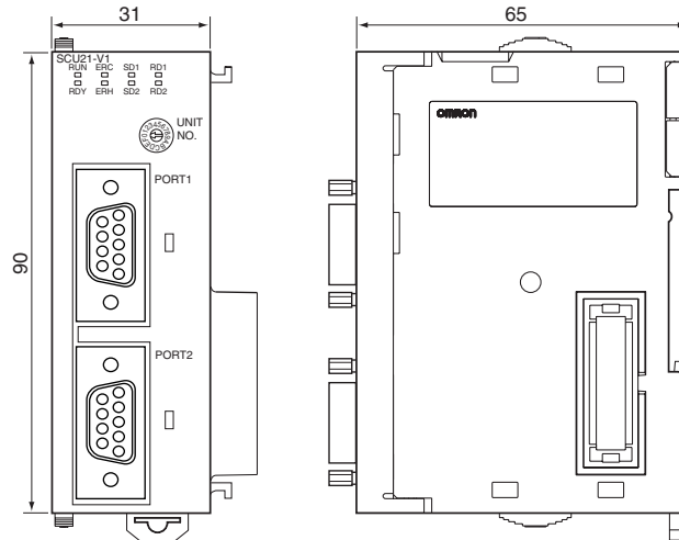
CJ1W-SCU31-V1
