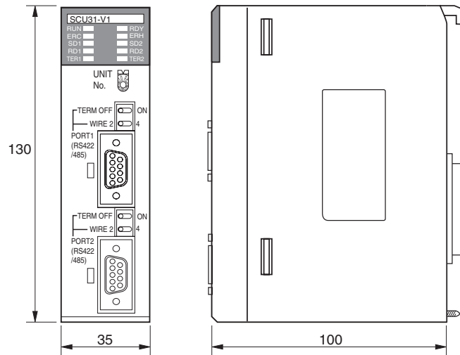
CS1W-SCU31-V1
