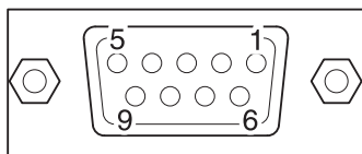
Разводка контактов гнезда DB9 (ПЛК)
