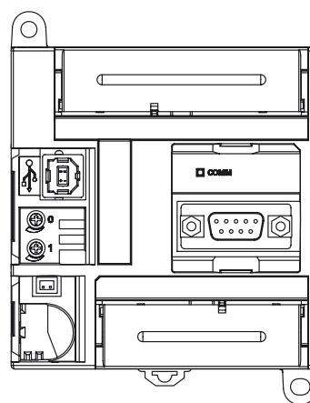
Модуль ЦПУ типа N CP1E-N20D□-□
